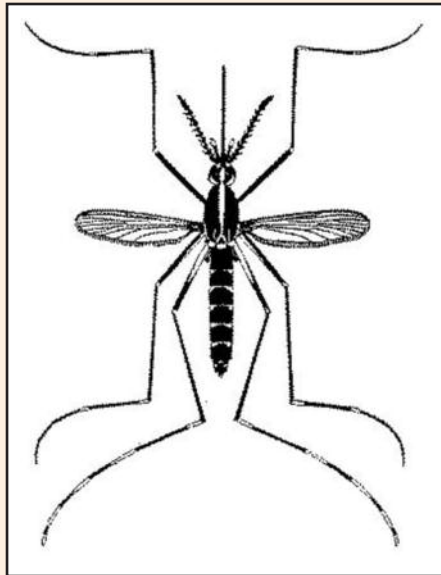
Aedes albopictus
