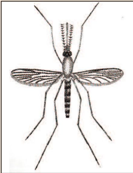
Culex pipiens
